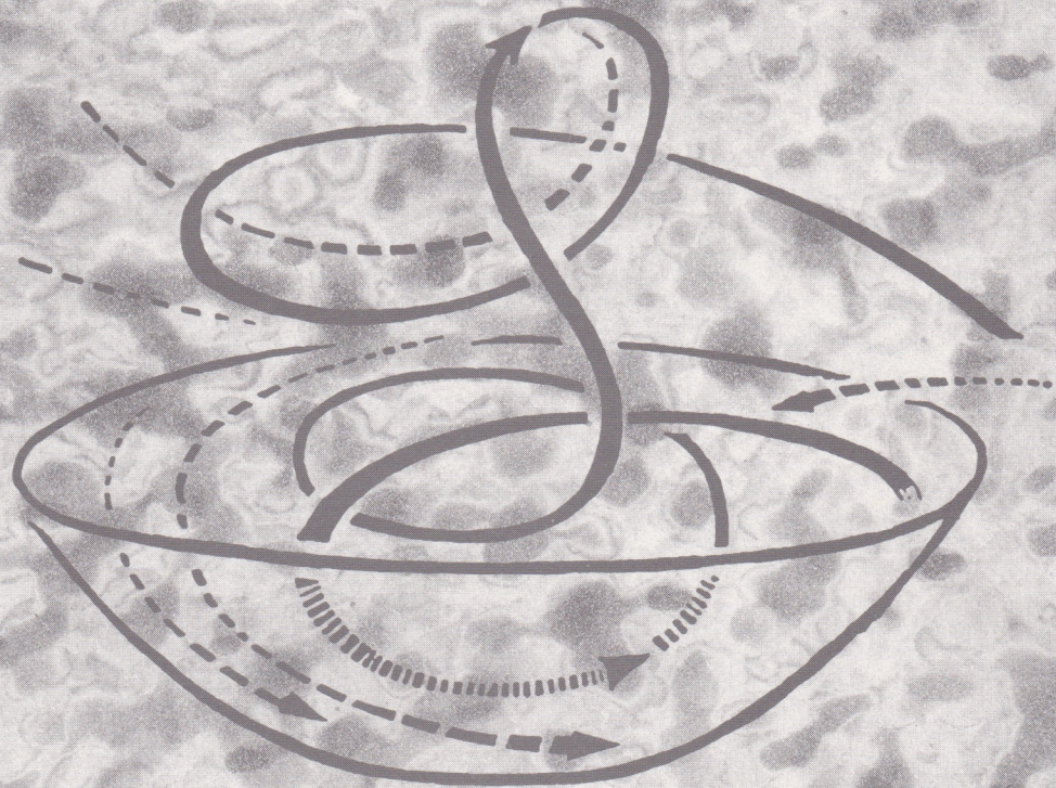
Wind in einem Tiefdruckgebiet (nach Blanc)
